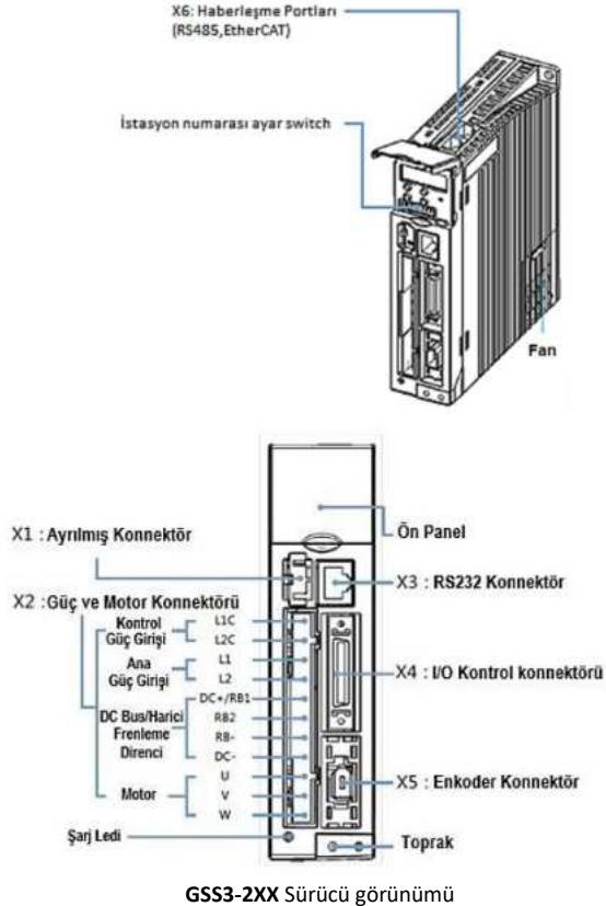
GSS3-2XX Sürücü görünümü
