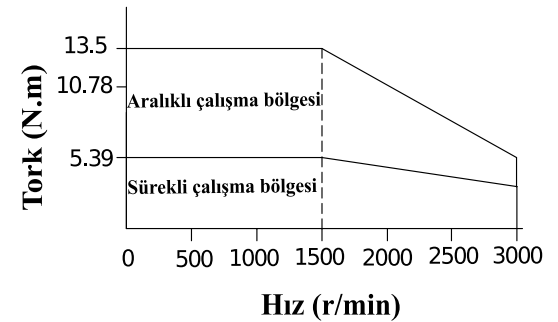
Tork - Hız Eğrisi
