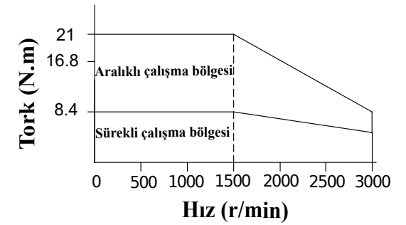
Tork - Hız Eğrisi
